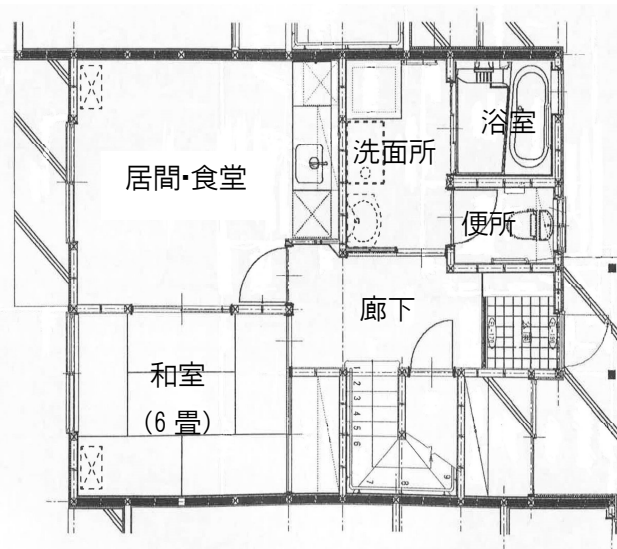
1階平面図
