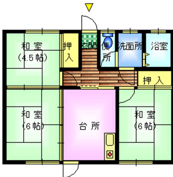
1階間取図
