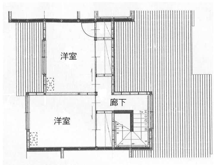
2階平面図
