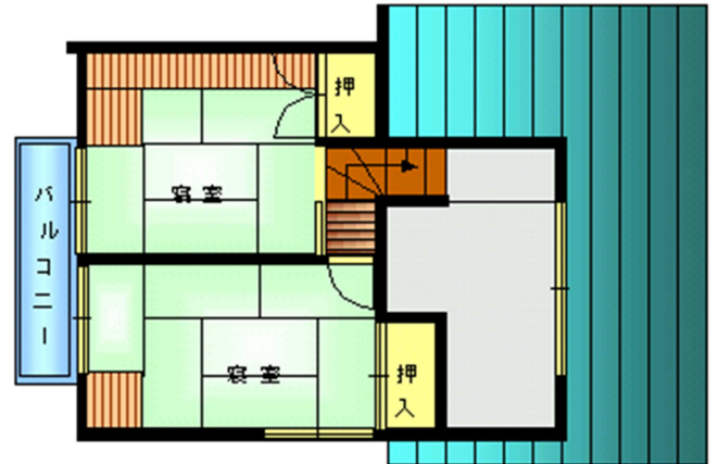
2階間取り図
