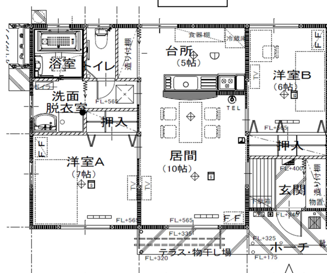
平面図
