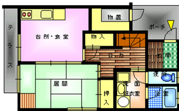
1 階間取図
